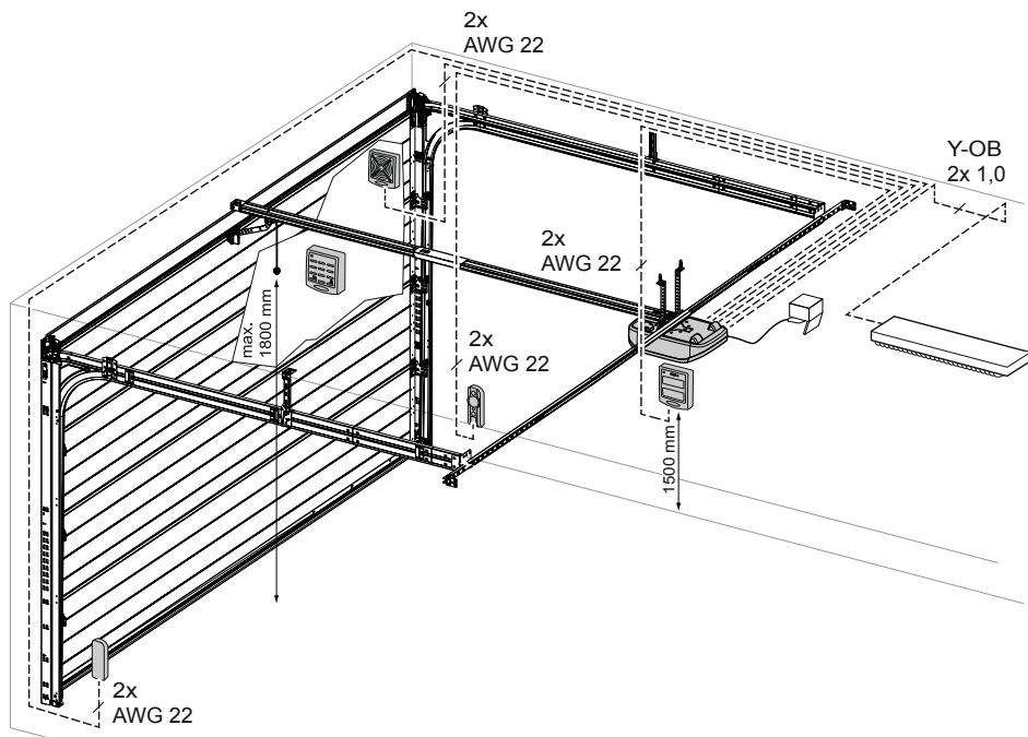
Afb. 3: Voorbeeldinstallatie accessoires
