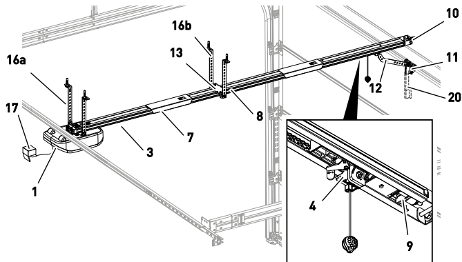
Afb. 1: Productoverzicht - opgebouwd
