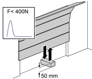
Afb. 7: Krachtbegrenzing controleren
