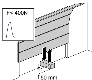
Afb. 7: Krachtbegrenzing controleren
